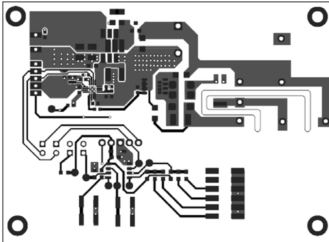
Figure 1—Top Layer
