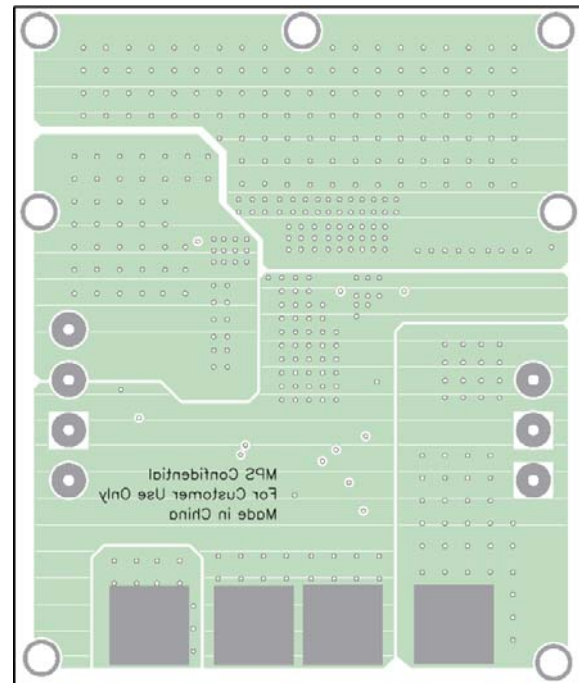
Figure 4—Bottom Layer
