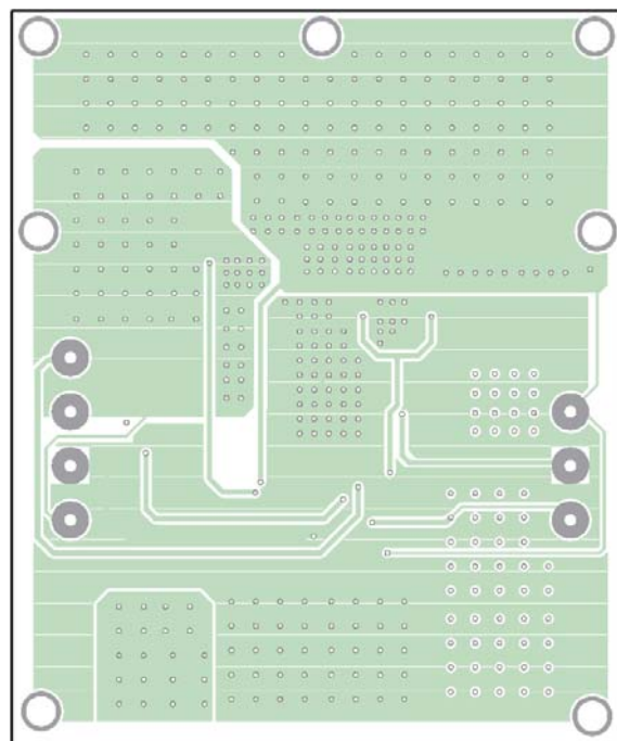
Figure 3—IN2 Layer
