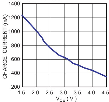
Thermal Protection ( V_{CE}=V_{IN}-V_{BAT} )
