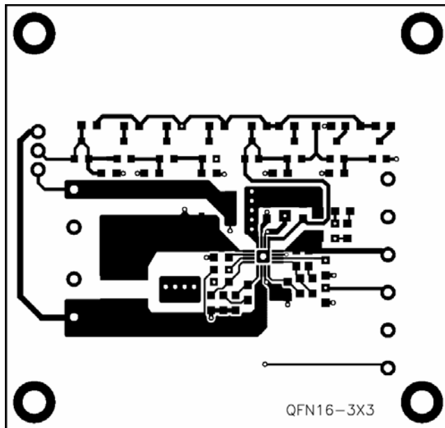
Figure 2—Top Layer
