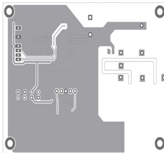
Figure 2—Bottom Layer
