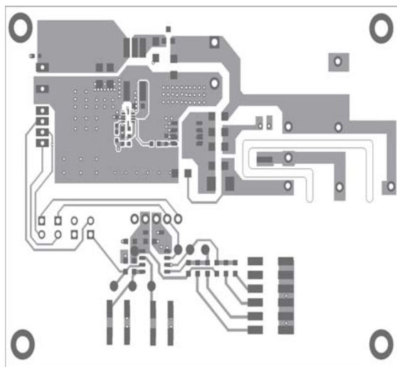
Figure 1—Top Layer
