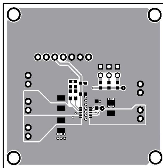
Figure 2—Top Layer
