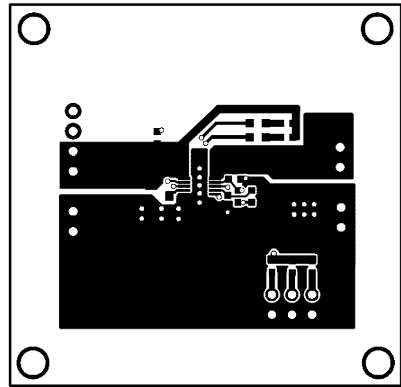
Figure 2—Top Layer
