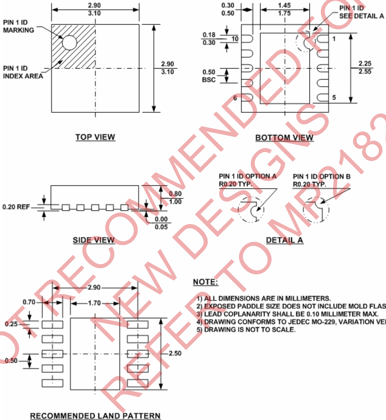
(3mmx3mm) QFN10
