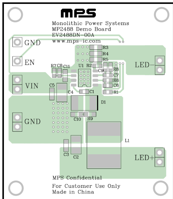
Figure 1—Top Layer
