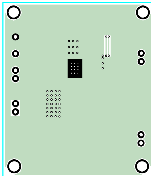
Figure 2—Bottom Layer
