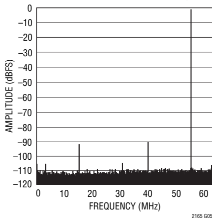
LTC2165 64k Point FFT, f_{IN} = 70\text{MHz} , -1\text{dBFS} , 125\text{Mpsps}
