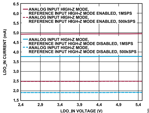
Figure 50. LDO_IN Current vs. LDO_IN Voltage, Internal LDO Enabled
