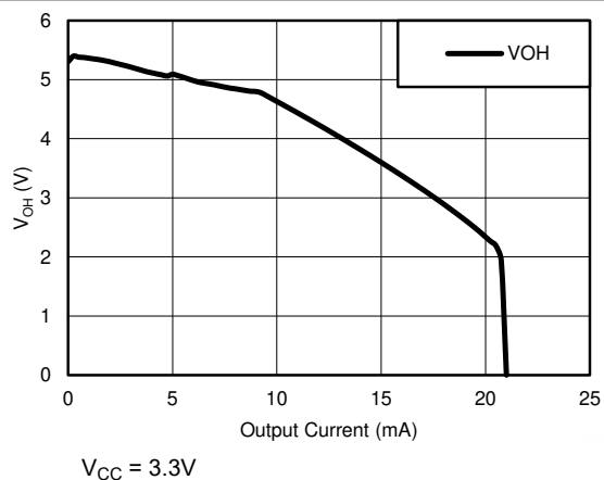
图 6-1. DOUT V_{OH} 与负载电流，两个驱动器均已加载
