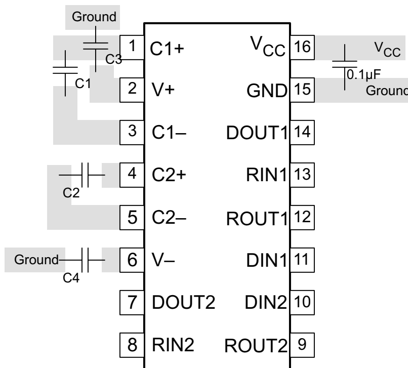
图 11-1. 布局图
