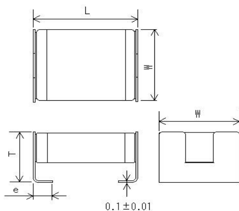
&lt; 1 chip type &gt;
