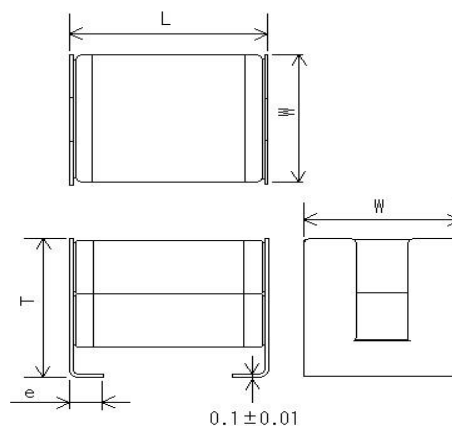
&lt; 2 chip type &gt;
