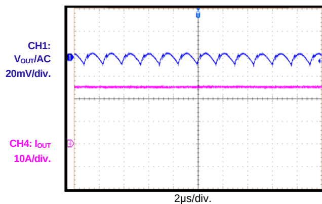
Ripple
