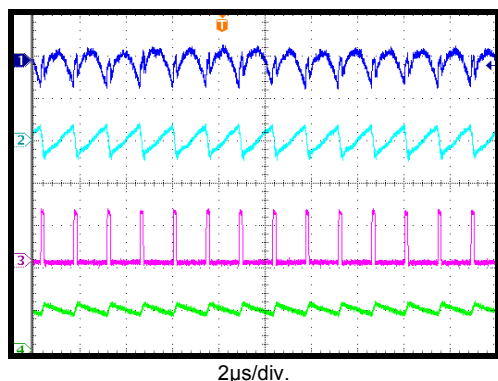
Input/Output Ripple
