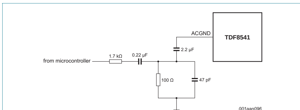
Fig 30. Beep input circuit
