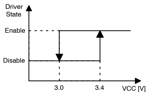
Figure 27. UVLO
